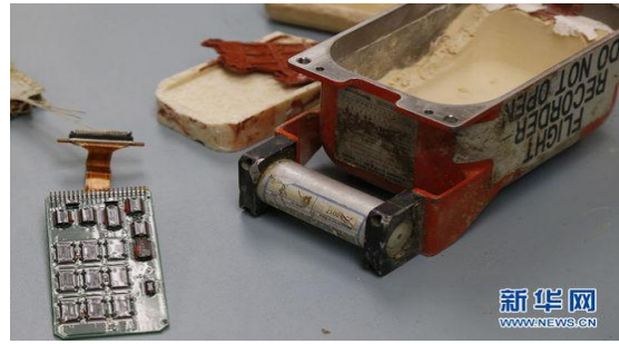
图为美国国家运输安全委员会的航空工程师打开放置飞行记录器芯片的部件
